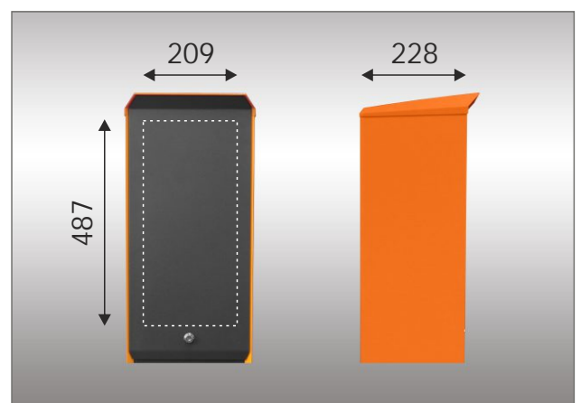
Einbaumaße Terminal MH
